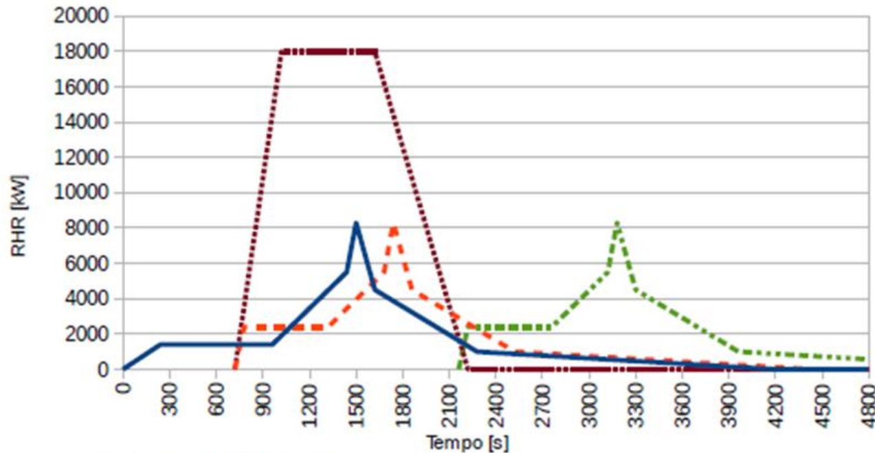
Illustrazione 24-1: Curve RHR(t) per lo scenario S3
